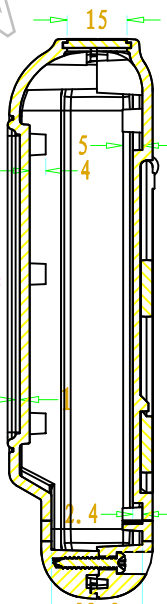
SEC A-A
